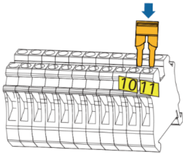
Terminale CA X3 dell'inverter (monofase)
