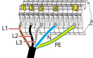
Terminale sul Backup Box (trifase)
